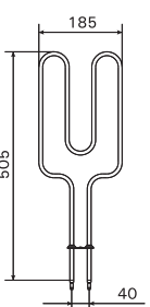
ZSA-420 250W/230V AV2, AV4, AV6
