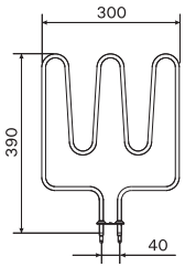
ZSK-690 1500W/230V KIP30/E, KIP45/E KV30/E, KV45/E KV50SE/A, M45/E V45/E
