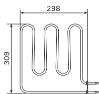
ZSB-224 1500W/230V BC45/E
