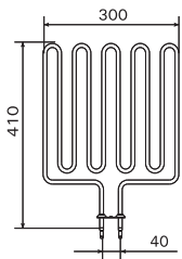
ZSL-318 3000W/240V L33
