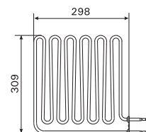
ZSB-229 3000W/230V BC90/E
