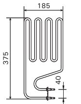
ZSJ-100 1000W/230V JM20/E, JM25/E
