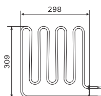
ZSB-226 2000W/230V BC60/E
