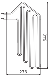
ZSF-30 2000W/230V AF6
