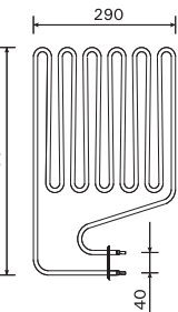
ZSP-255 3000W/230V F16,5, F18 K11G/S PO165
