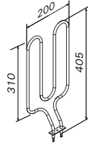
ZSN-150 1150W/230V D23/E, D23EE, D29EE
