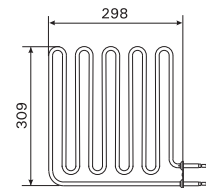
ZSB-228 2670W/230V BC80/E
