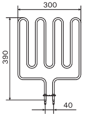
ZSK-700 2000W/230V KIP60/E KV60/E, M60/E, KV60SE/A, V60/E
