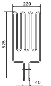
ZSA-430 1900W/230V AV2, AV4, AV6
